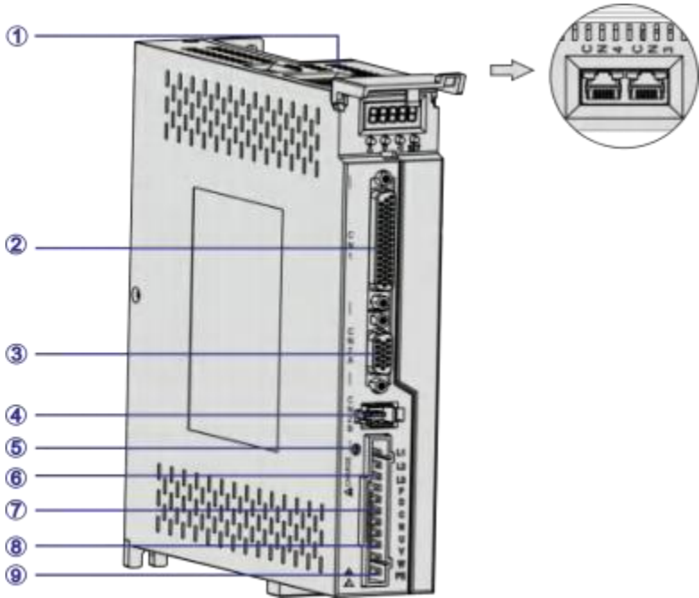
图 1.1 ECX-30伺服驱动器前面板介绍
