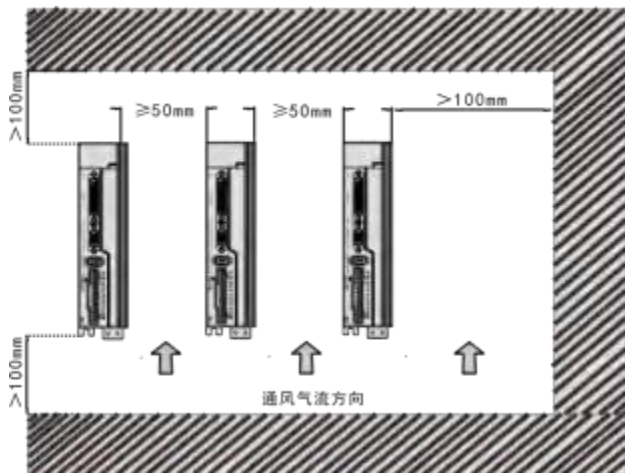
图 1.3 安装间隔
