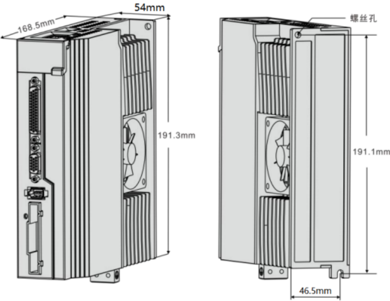
图 3.1 ECX-30系列外形尺寸图
