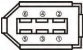
图4.8 CN2B编码器信号端子
