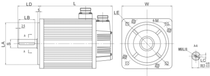
图 3.3 130 电机和表 3-2
